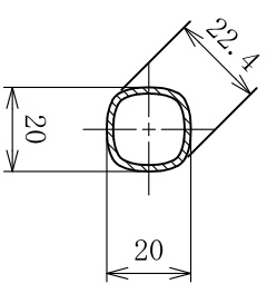
B-B断面図
